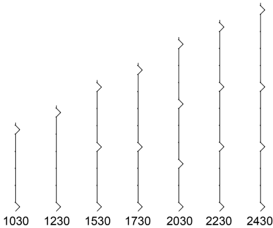
PRZEKRÓJ PANELI PRZETŁACZANYCH
